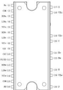
PIN1-PIN25
